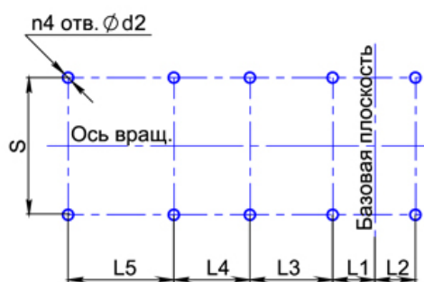
Схема расположения отверстий для крепления вентилятора
