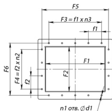
Вид Е
