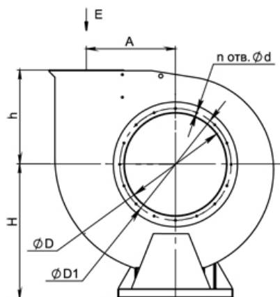
Вид Е
