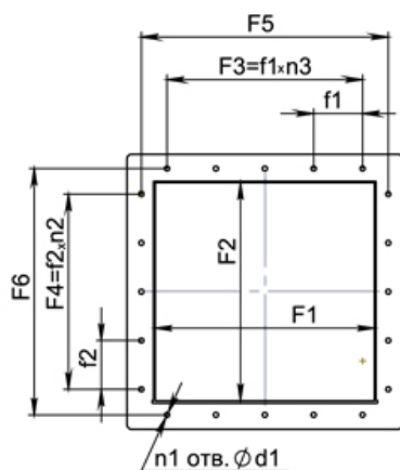
Вид Е
