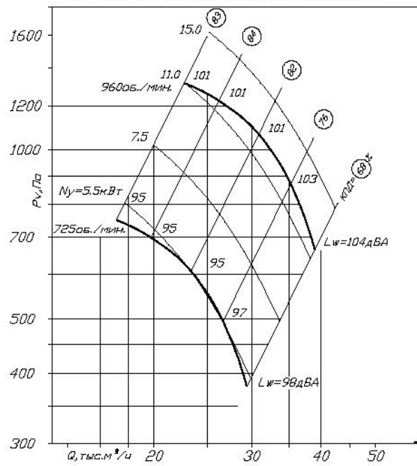
BP 80-75-10 D=0.95D_{\text{ном}} схема 1
