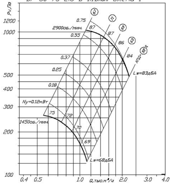
БР 80-75-2.5 D=1.1D_{ном} схема 1
