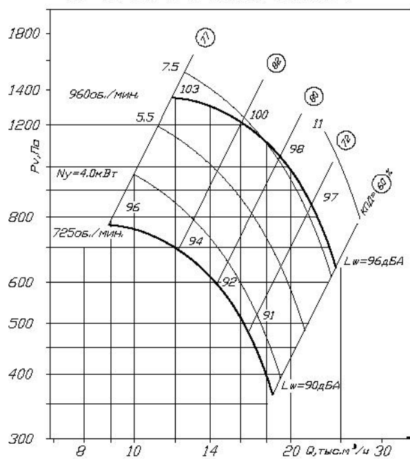
БР 80-75-8 D=1.1D_{ном} схема 1
