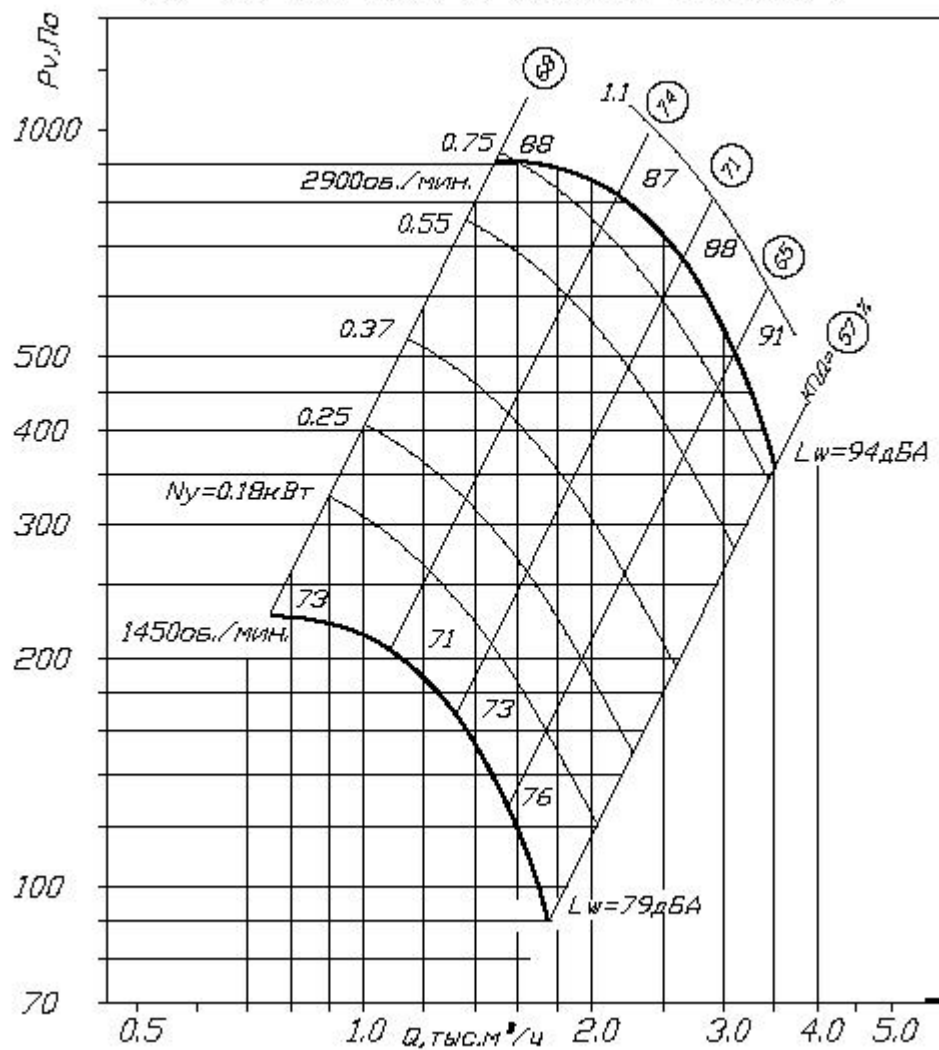
БР 80-75-3.15 D=0.9D_{\text{ном}} схема 1
