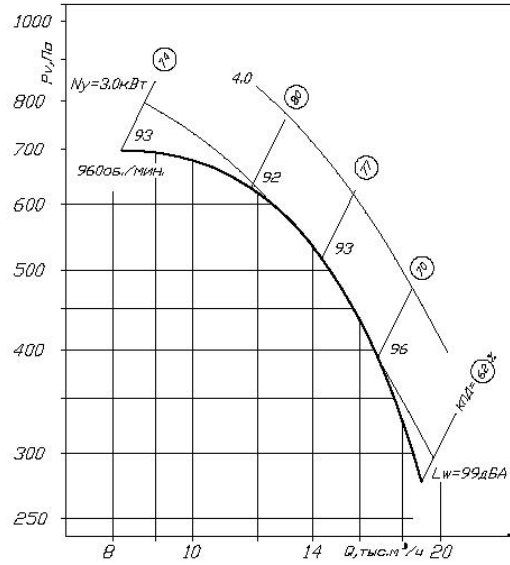
BP 80-75-8 D=0,9D_{\text{ном}} схема 1
