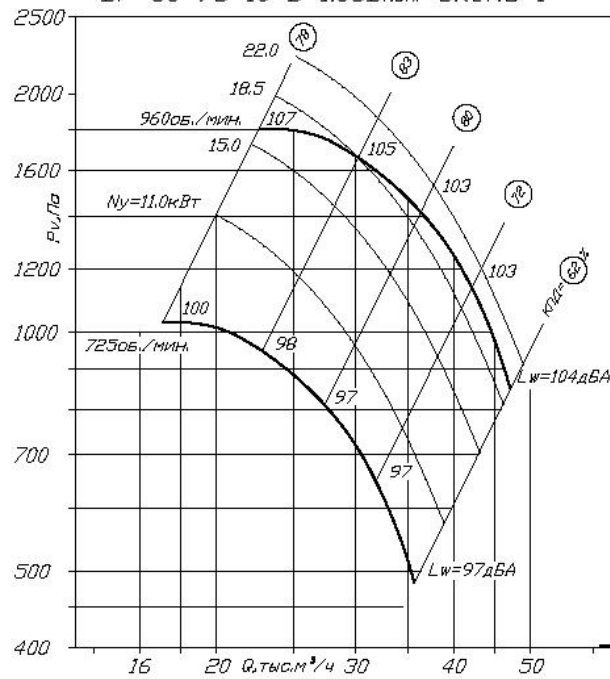
BP 80-75-10 D=1.05D_{\text{ном}} схема 1
