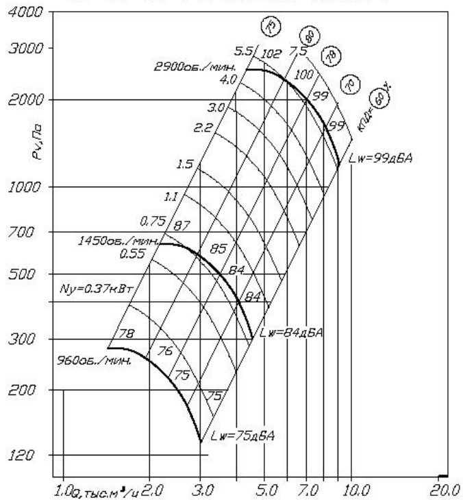
BP 80-75-4 D=1.05D_{\text{ном}} схема 1
