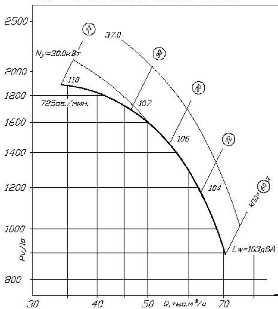
БР 80-75-12.5 D=1.1D_{\text{ном}} схема 1
