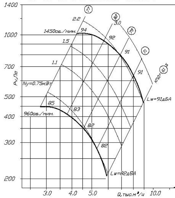
BP 80-75-5 D=1.05D_{\text{ном}} схема 1
