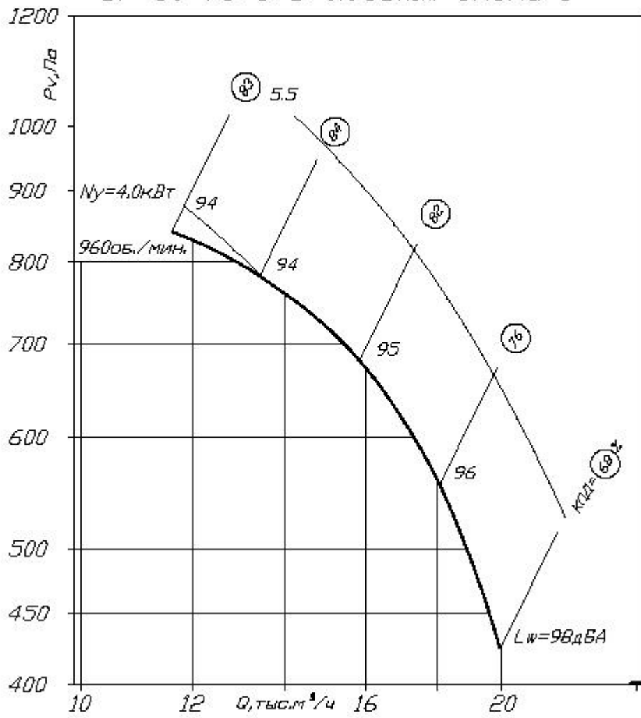
BP 80-75-8 D=0,95D_{\text{ном}} схема 1
