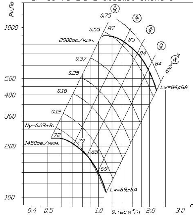
БР 80-75-2.5 D=1.05D_{ном} схема 1
