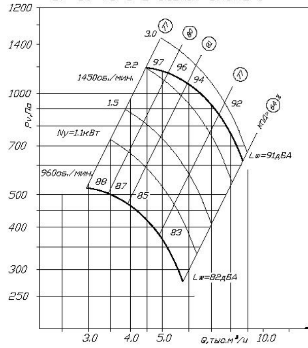
BP 80-75-5 D=1.1D ном схема 1
