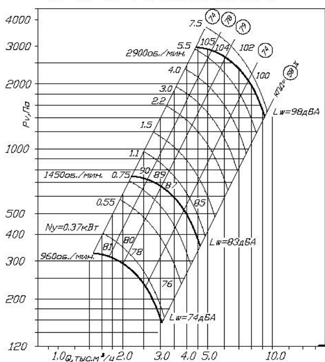
BP 80-75-4 D=1.1D_{\text{ном}} схема 1
