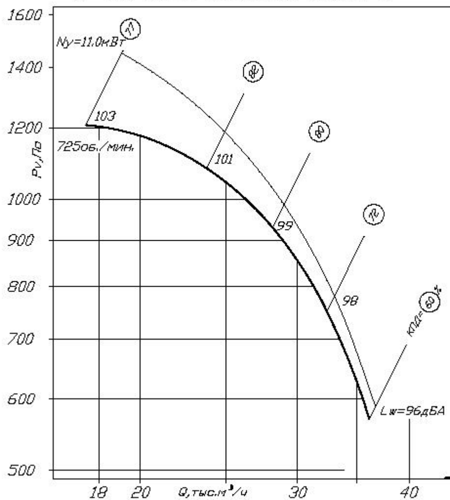
БР 80-75-10 D=1.1D_{\text{ном}} схема 1
