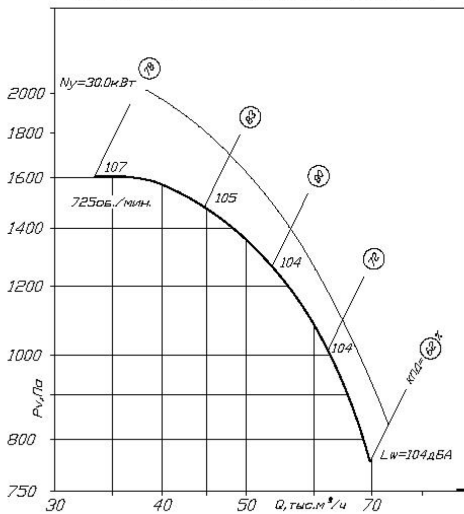
BP 80-75-12.5 D=1.05D_{\text{ном}} схема 1
