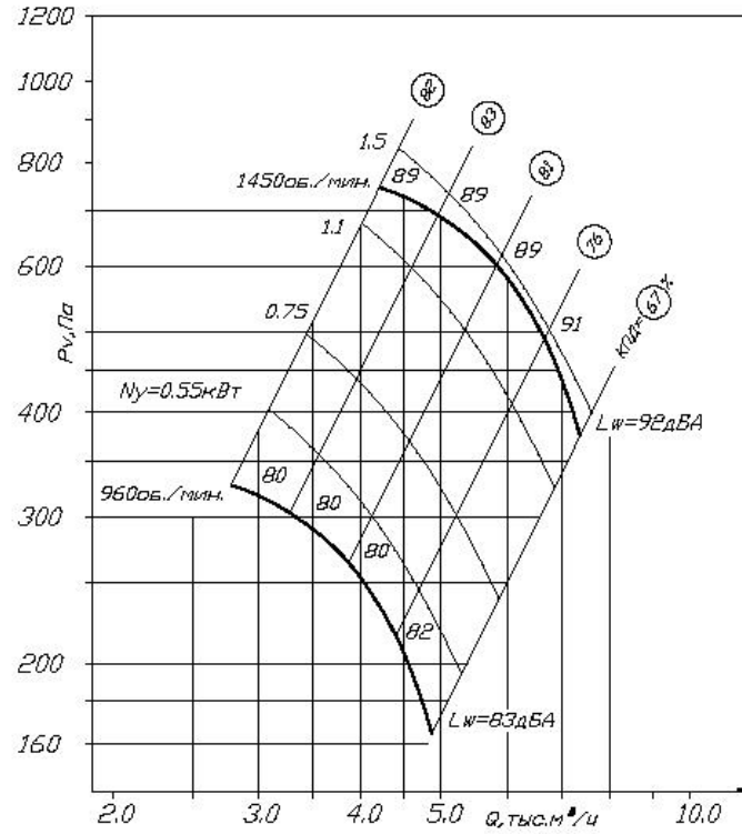
BP 80-75-5 D=0.95D_{\text{ном}} схема 1
