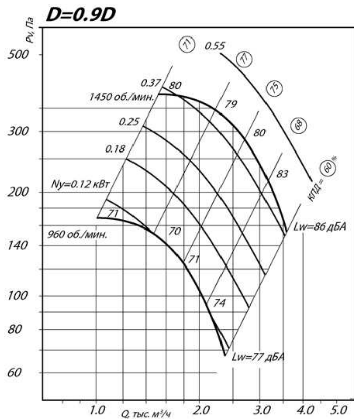
Аэродинамические характеристики вентилятора ВР 86-77 №4 схема 1
