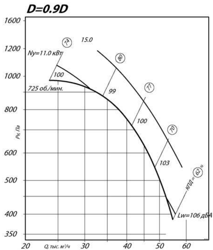
Аэродинамические характеристики вентилятора ВР 86-77 №12,5 схема 1
