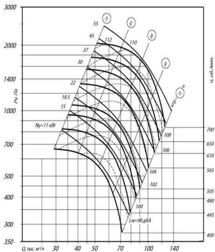
Аэродинамические характеристики вентилятора ВР 86-77 №16 схема 1
