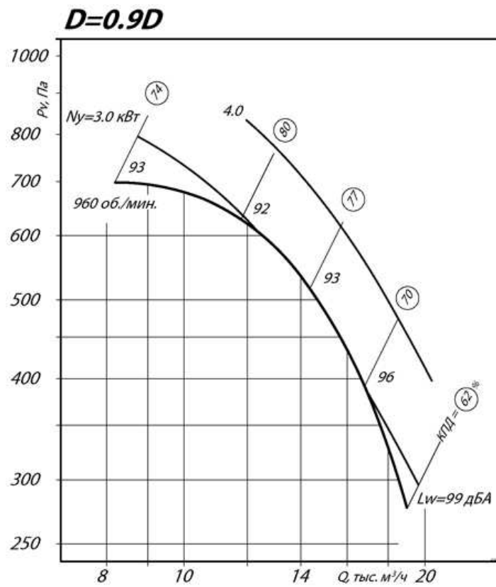
Аэродинамические характеристики вентилятора ВР 86-77 №8 схема 1, схема 5
