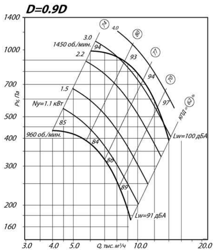
Аэродинамические характеристики вентилятора ВР 86-77 №6,3 схема 1
